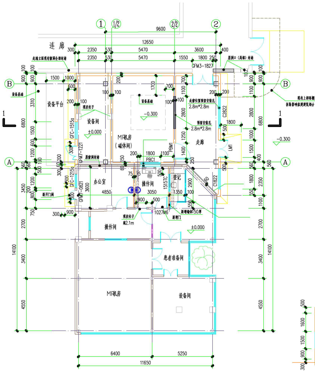
首层平面图 1:100
